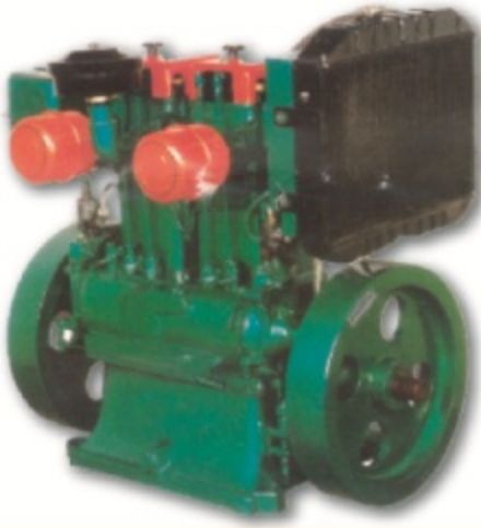
Moteurs diesel de 20 CV Modèle type Lister
